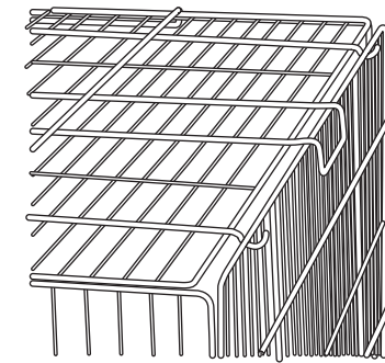
天井パネルの引っ掛けフック部
