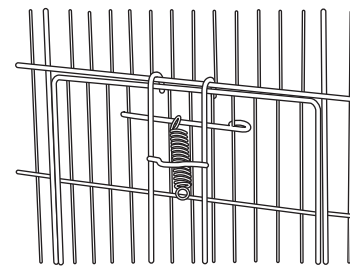
天井パネルの引っ掛けフック部
